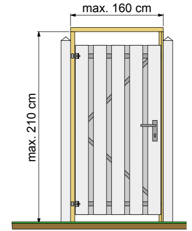
Universeel tuindeurkozijn
